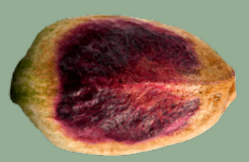
Kernel
